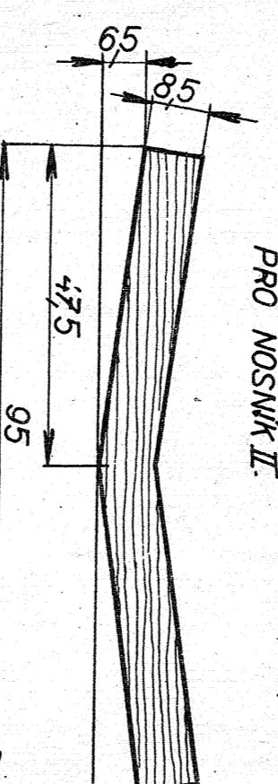
SPUJ KŘÍDEL - PŘEKL. 3mm (NEB 3x1mm) PRO NOSNÍK II
