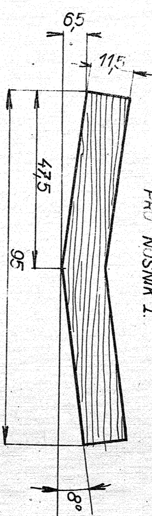
SPUJ KŘÍDEL - PŘEKL. 5mm (NEB 5x1mm) PRO NOSNÍK I
